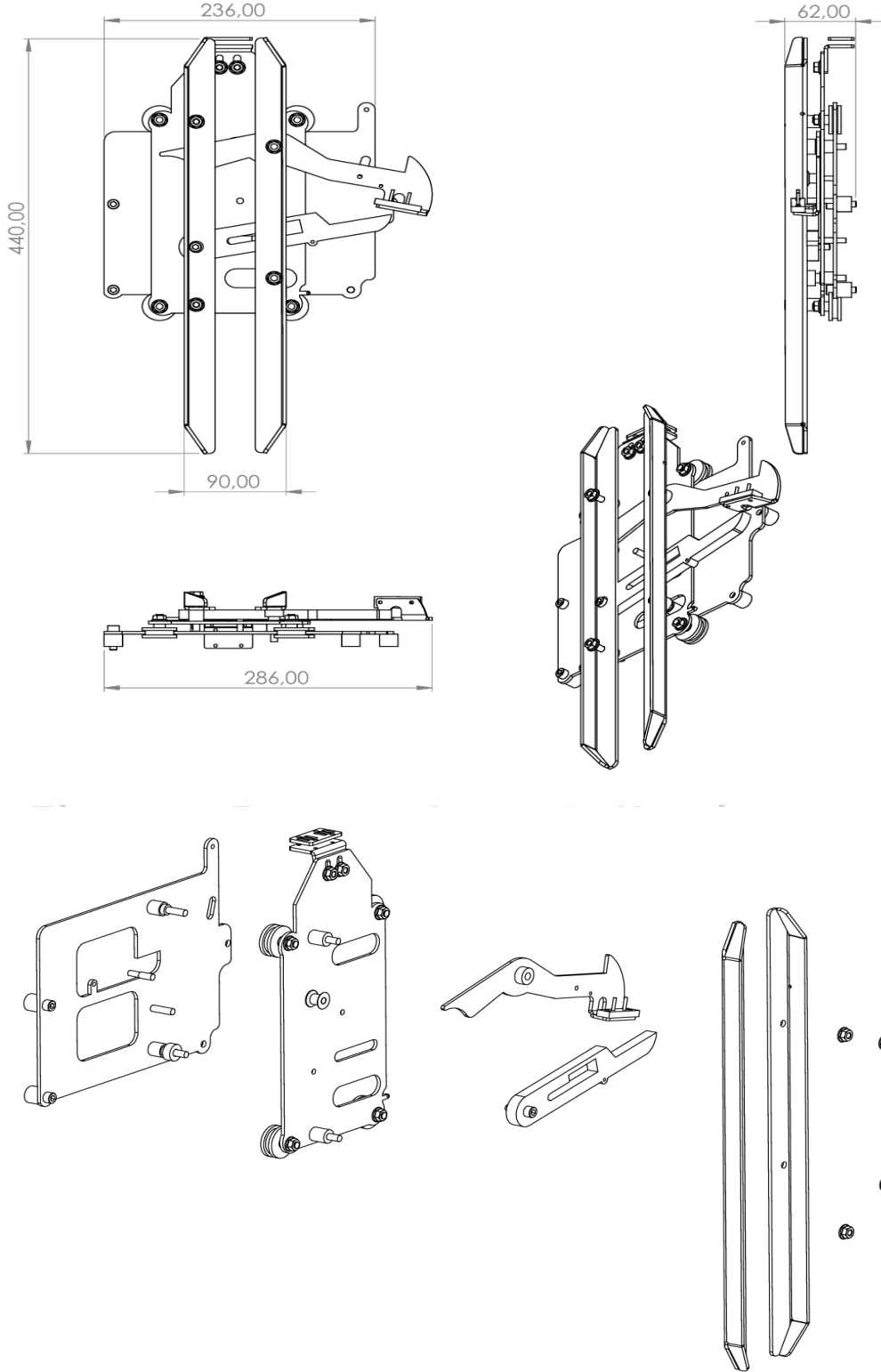
Şekil-1.2 81-20 Kaşık Detay
